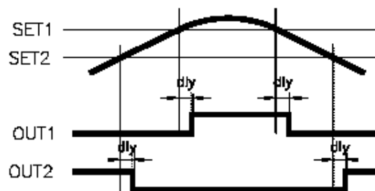
Retardo por temporización para OUT1 en modo HI y OUT2 en modo LO
