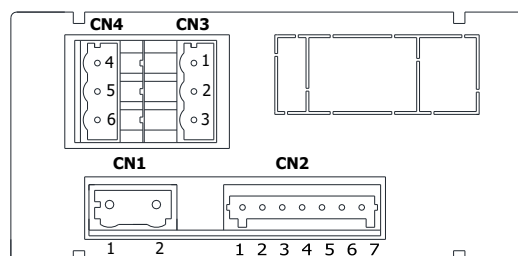
Localización de los conectores posteriores.
