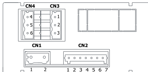
Agencement des connecteurs postérieurs.
